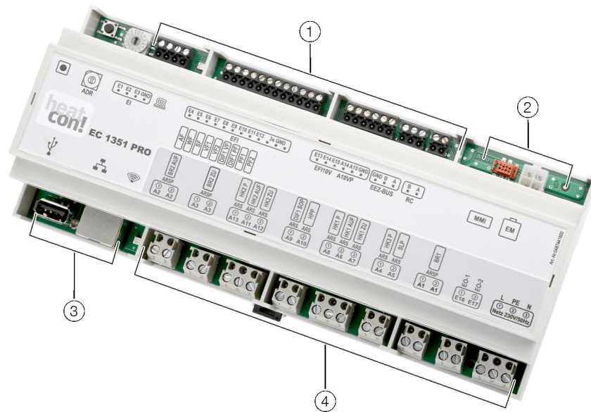
Fig. 3: heatcon! EC
